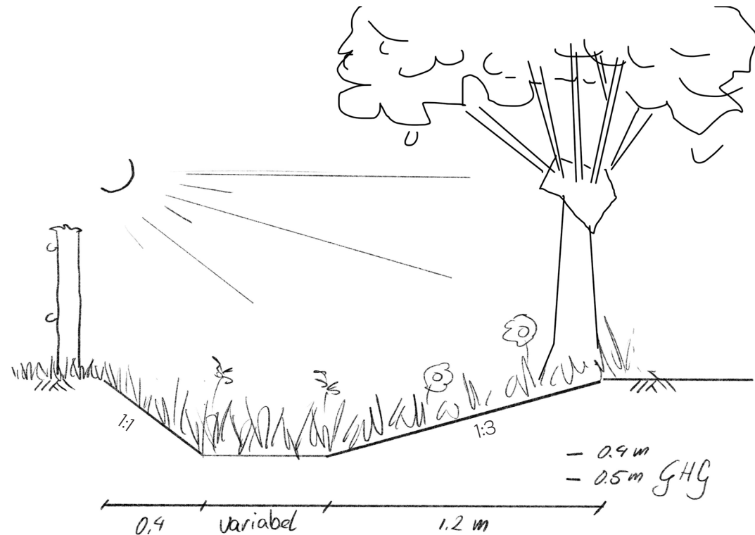
Principeprofiel infiltratiegreppel
