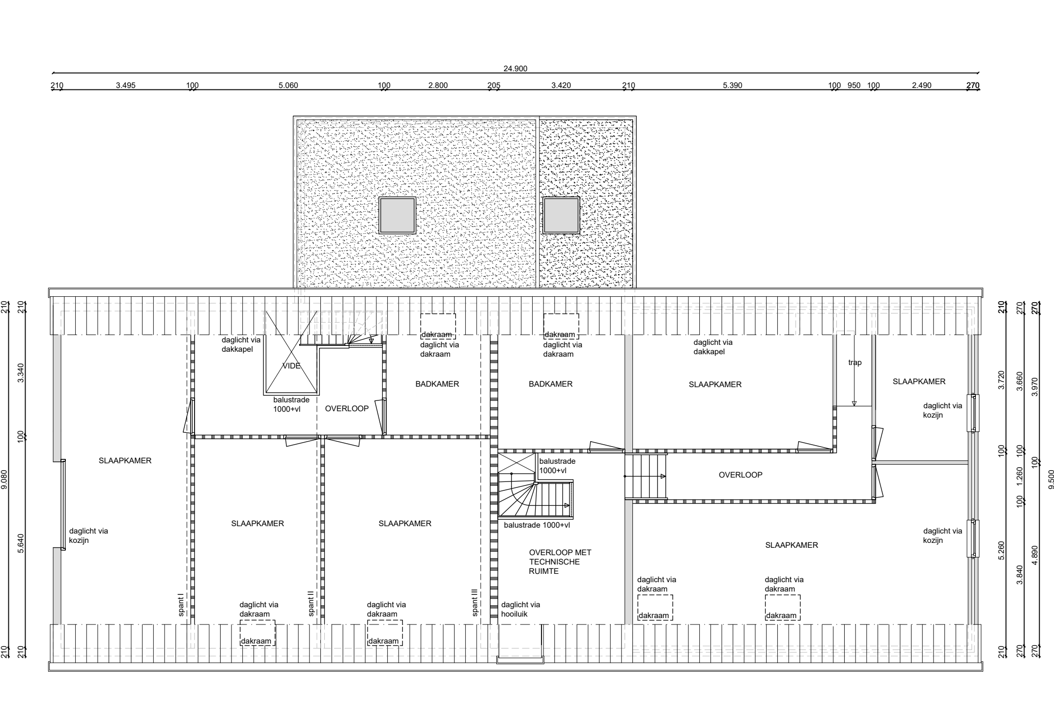
VERDIEPING - renovatie
