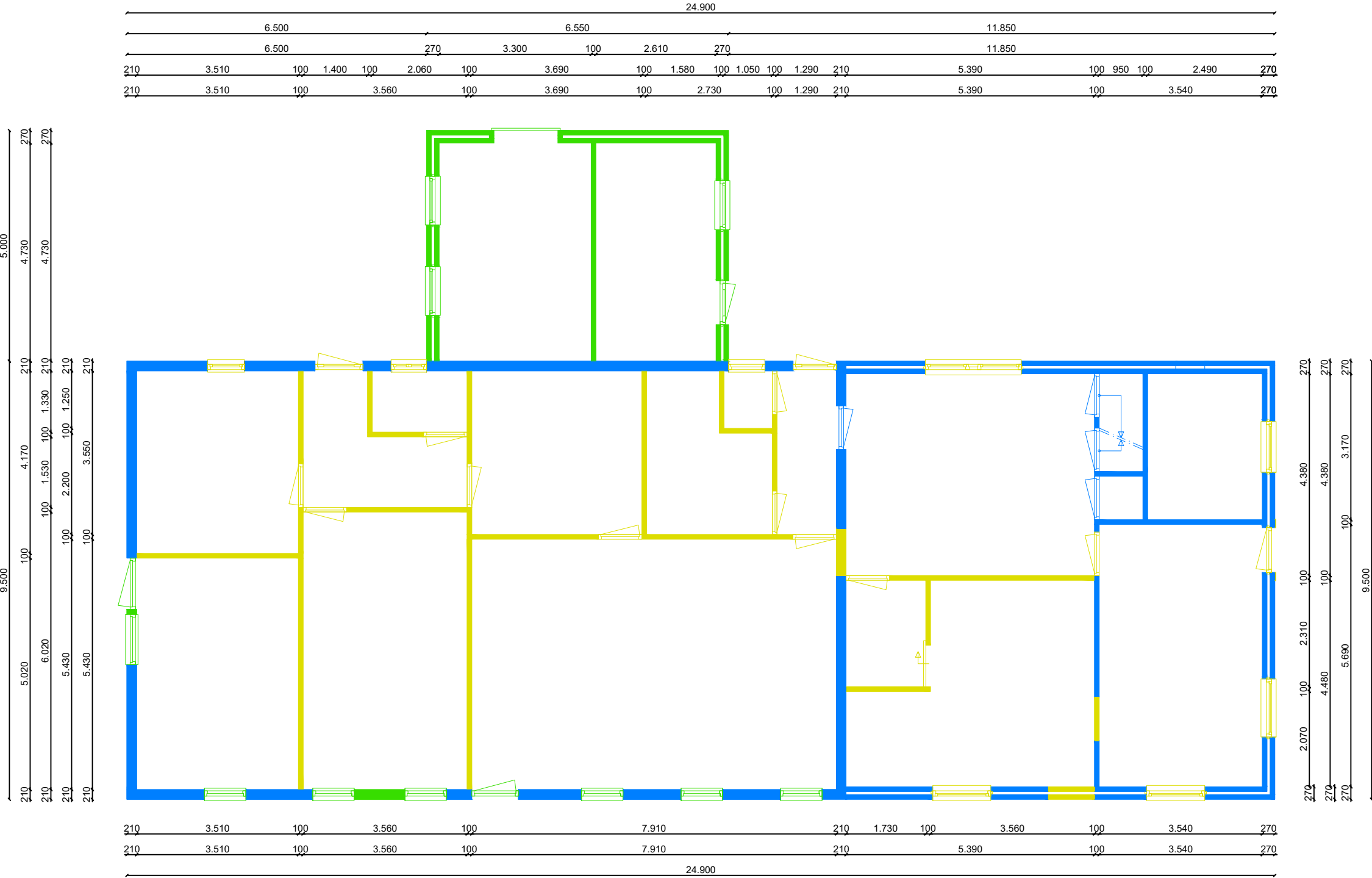
BEGANE GROND - waarderingstekening
