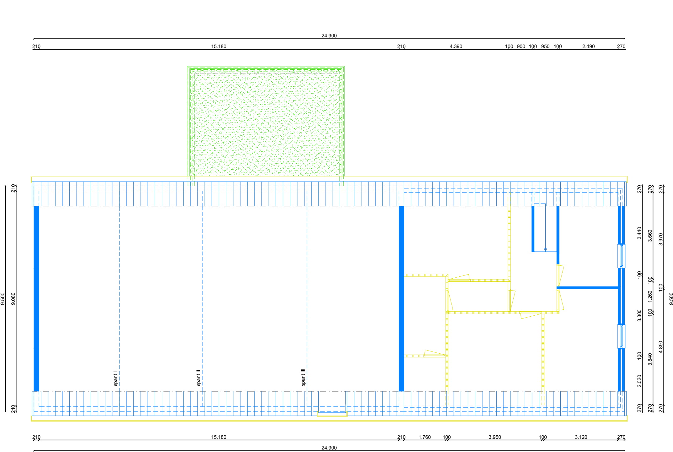
VERDIEPING - waarderingstekening
