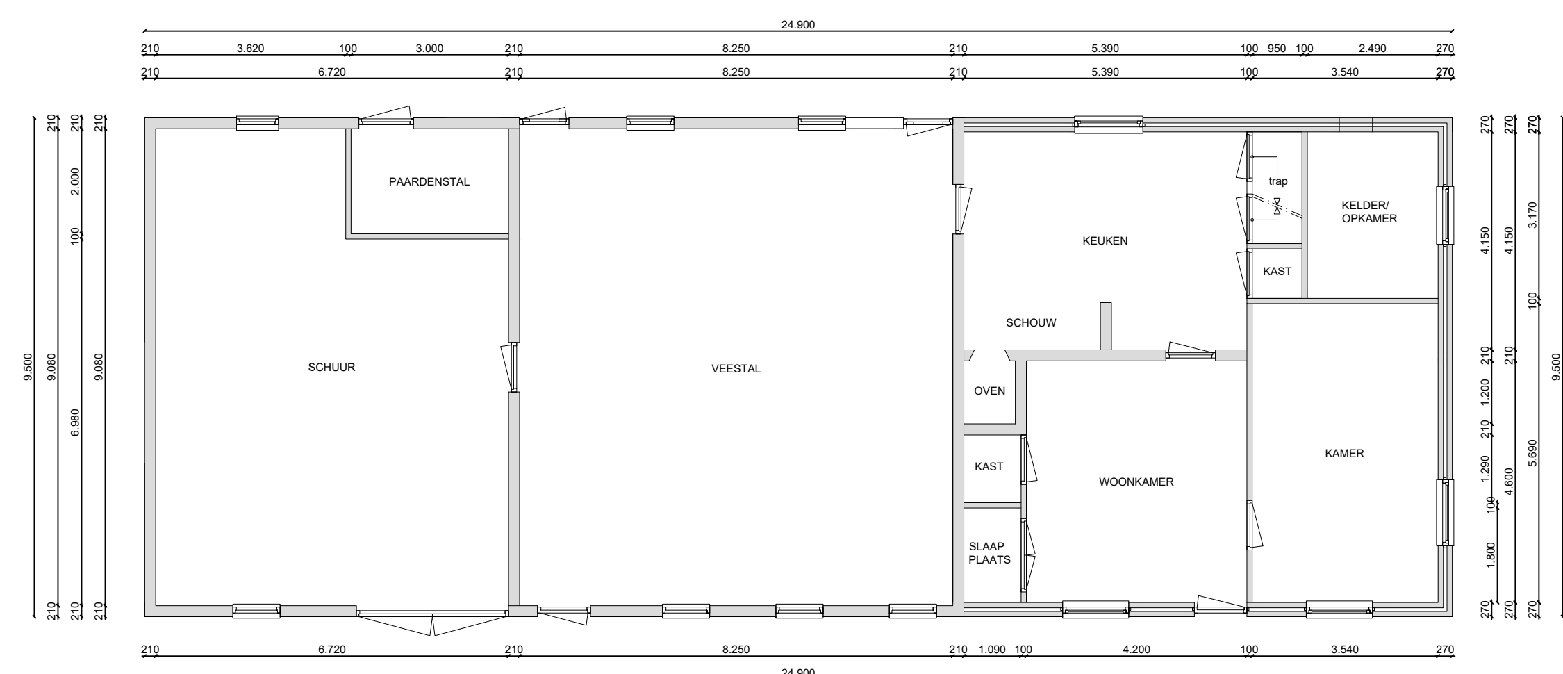
BEGANE GROND - oorspronkelijke situatie 1932
