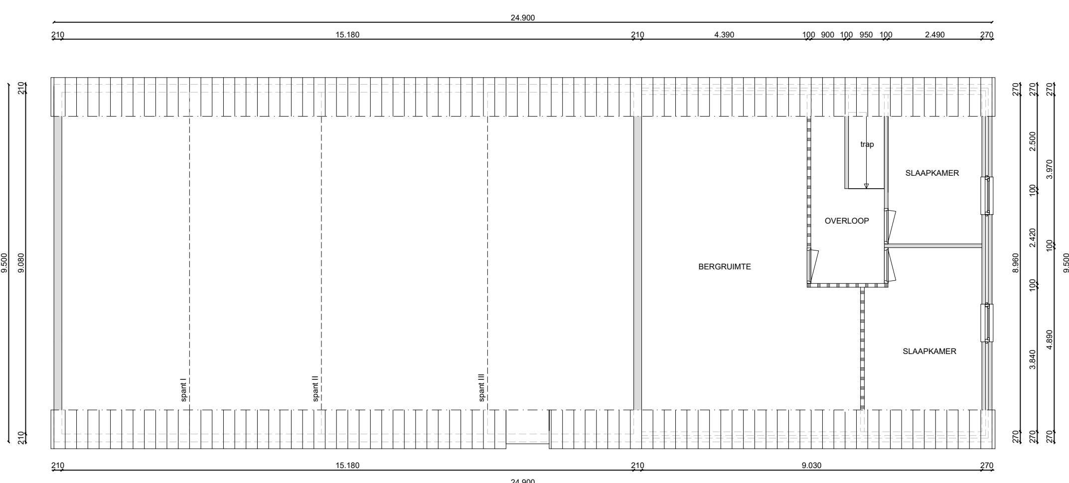
VERDIEPING - oorspronkelijke situatie 1932
