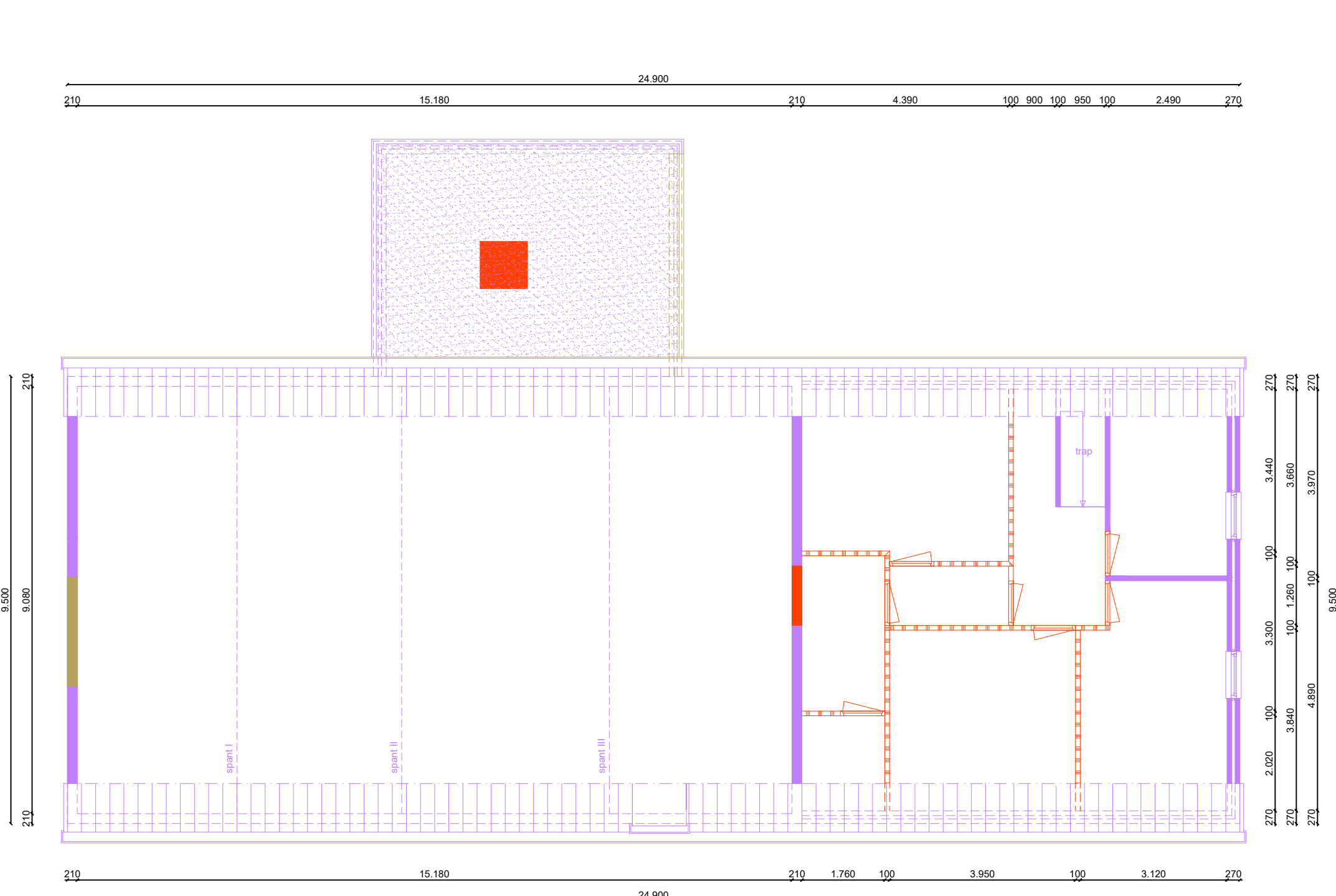
VERDIEPING - slooptekening
