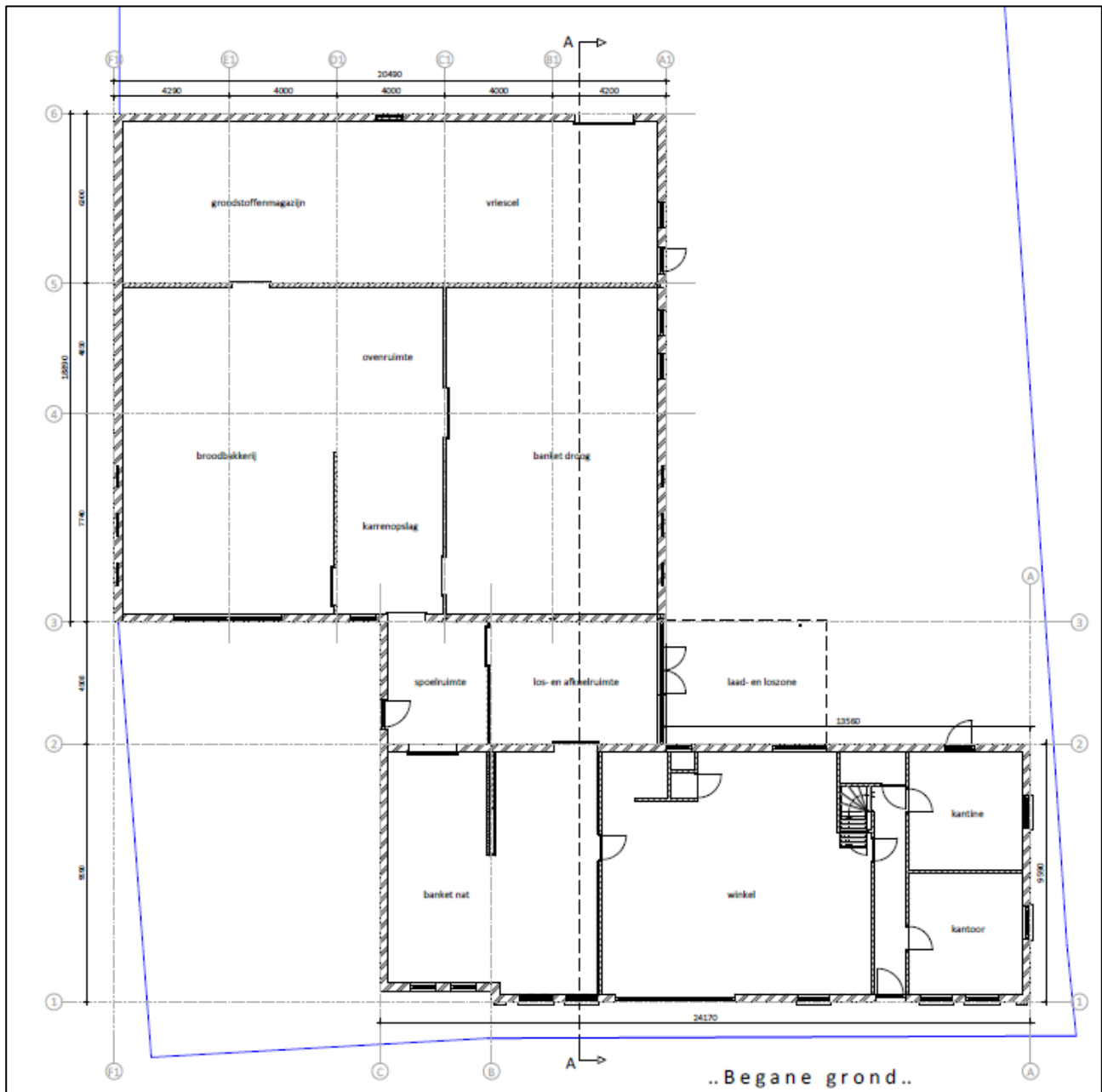
Afbeelding 1: plattegrondtekening begane grond bestaande situatie
