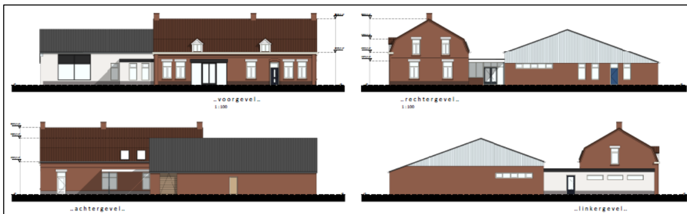
Afbeelding 3: gevelaanzichten bestaande situatie
