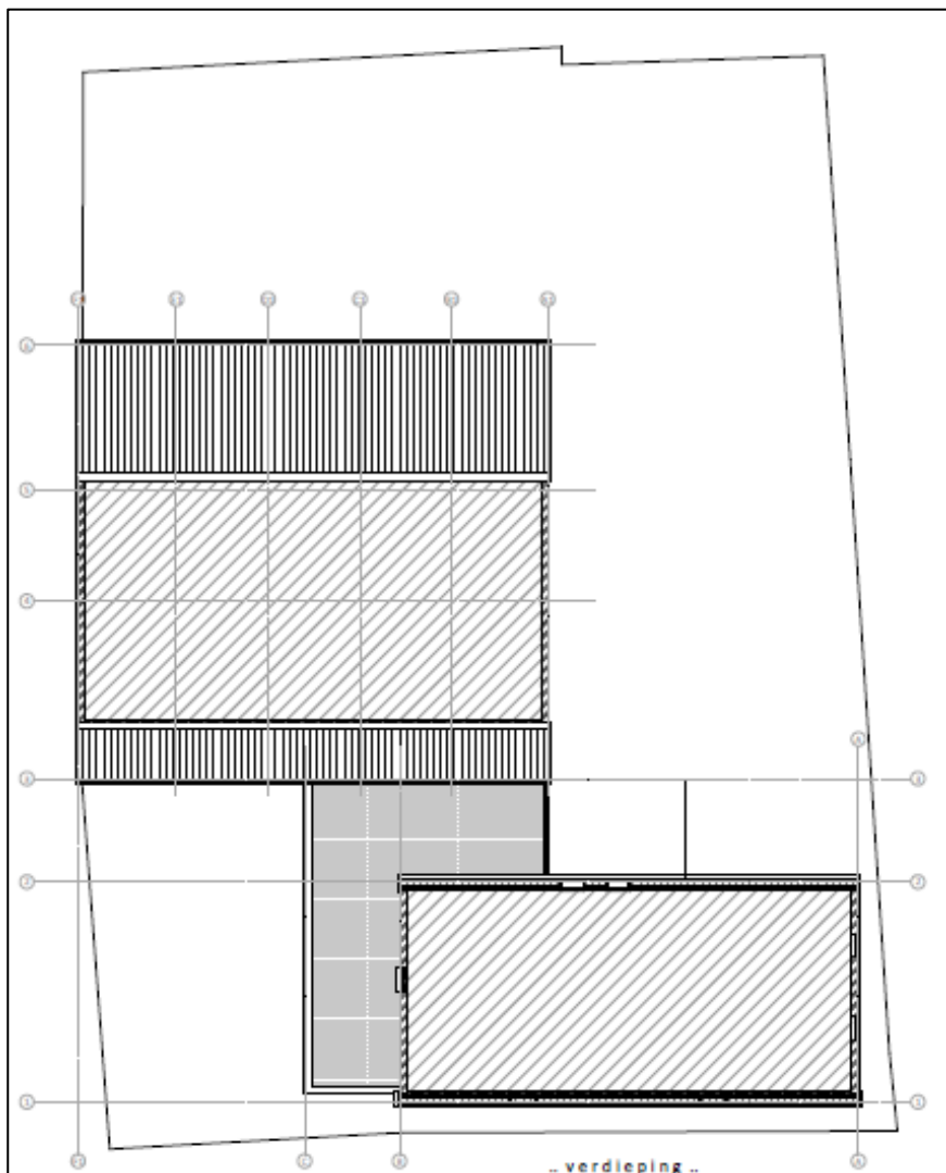
Afbeelding 2: plattegrondtekening verdieping bestaande situatie
