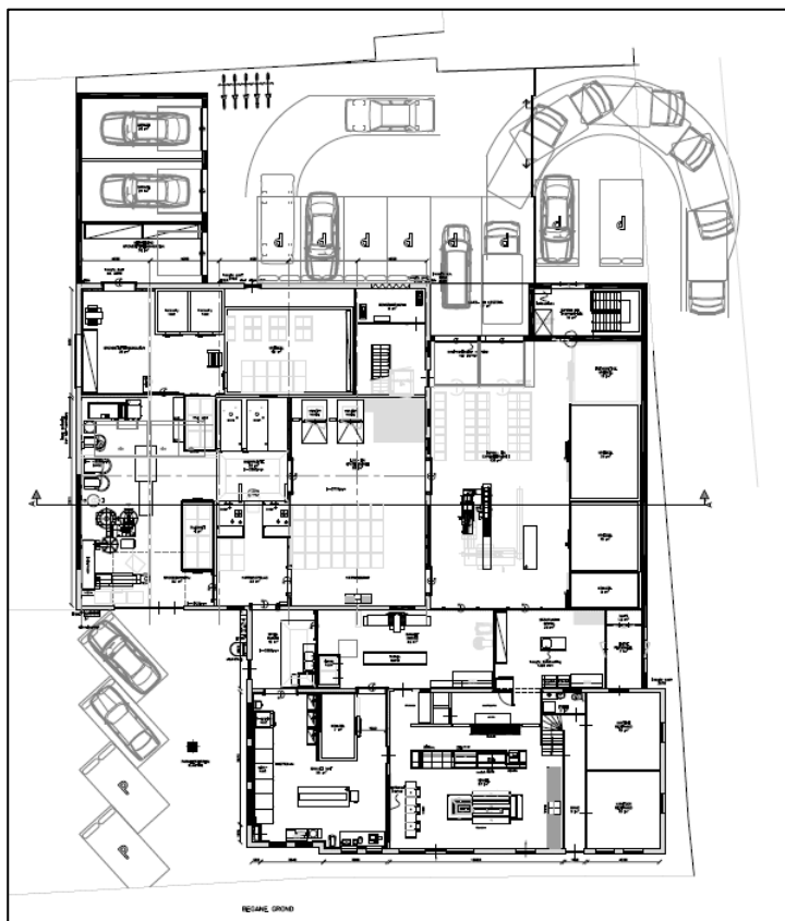
Afbeelding 4: plattegrondtekening begane grond beoogde situatie
