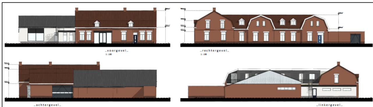
Afbeelding 6: gevelaanzichten beoogde situatie
